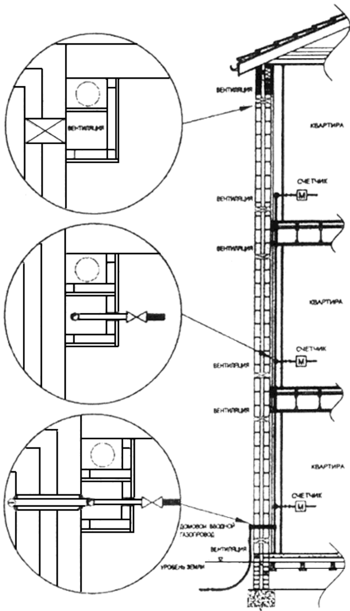
Рисунок Г.1 - Газопровод в вентилируемой штрабе
