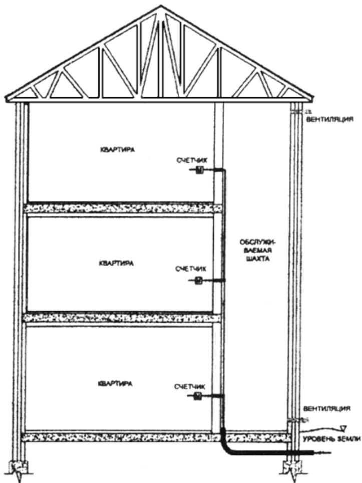
Рисунок Г.2 - Газопровод в вентилируемой шахте
